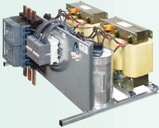
Moduleinschub MDL75 100/2LD4 14% Verdrosselung Schutzart IP 00
